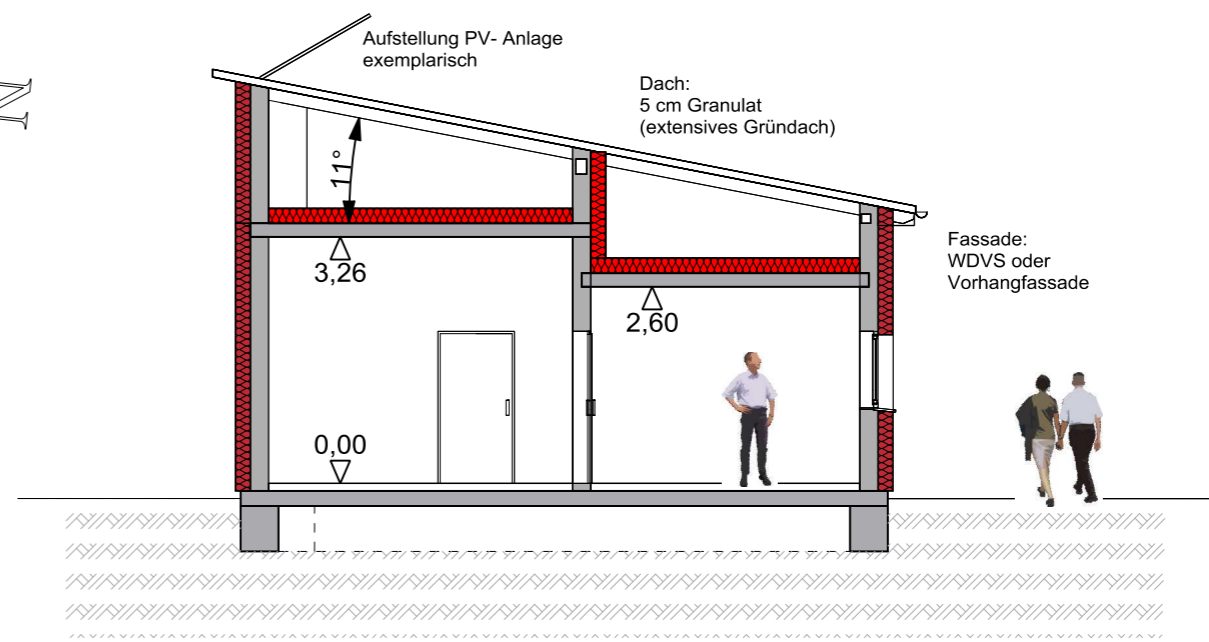
SCHNITT A-A
